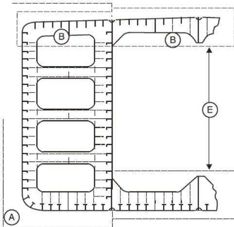
Petrolero: sección transversal típica
