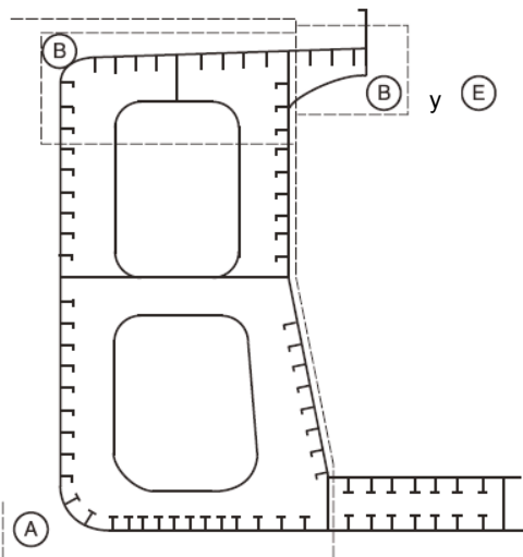
Mineralero/petrolero: sección transversal típica
