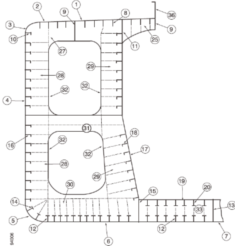
Sección transversal típica de un mineralero/petrolero en la que se indican los miembros longitudinales y transversales
