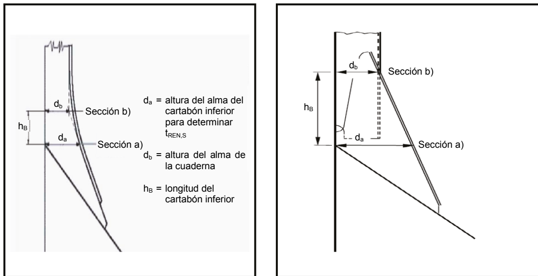
Figura 4 – Secciones a) y b)
