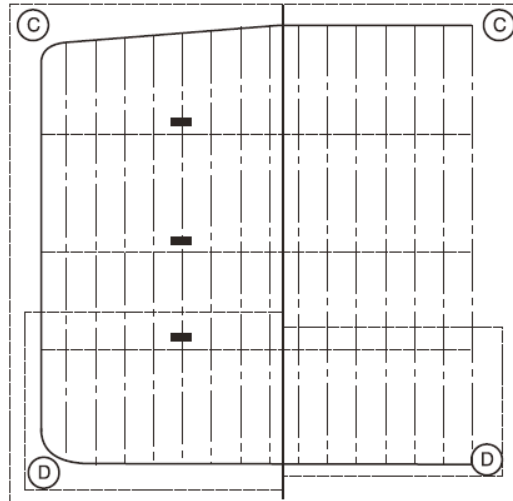
Petrolero: mamparo transversal típico
