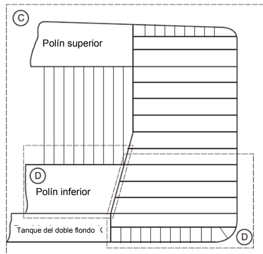
Mineralero/petrolero: mamparo transversal típico
