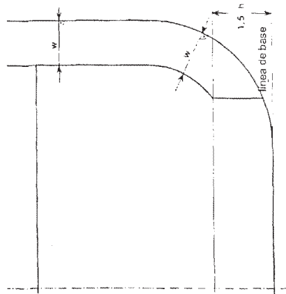
Figura 2 - Definición de los límites de los tanques de carga a efectos del párrafo 4 de la presente regla
