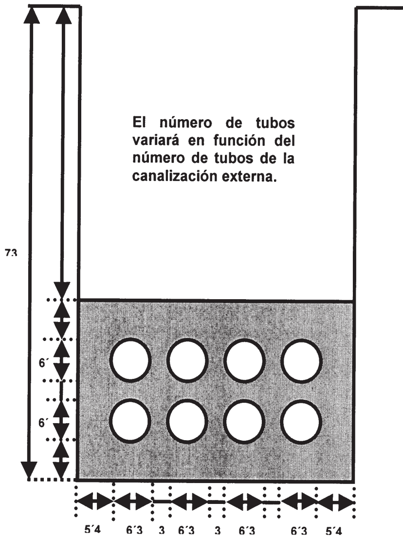
APÉNDICE 4: EJEMPLO DE SECCIÓN TRANSVERSAL DE CANALIZACIÓN DE ENLACE SUBTERRANEA DE 8 TUBOS.
