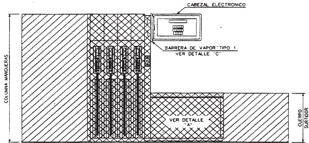
ALZADO
