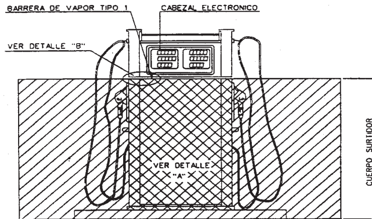
ALZADO
