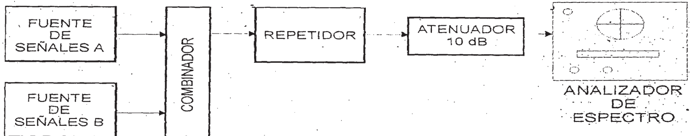
Figura 6: Montaje de medida para la atenuación de intermodulación (dos señales de entrada)
