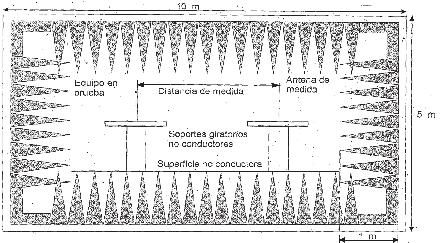
Figura 2: Especificación para el apantallamiento y las reflexiones
