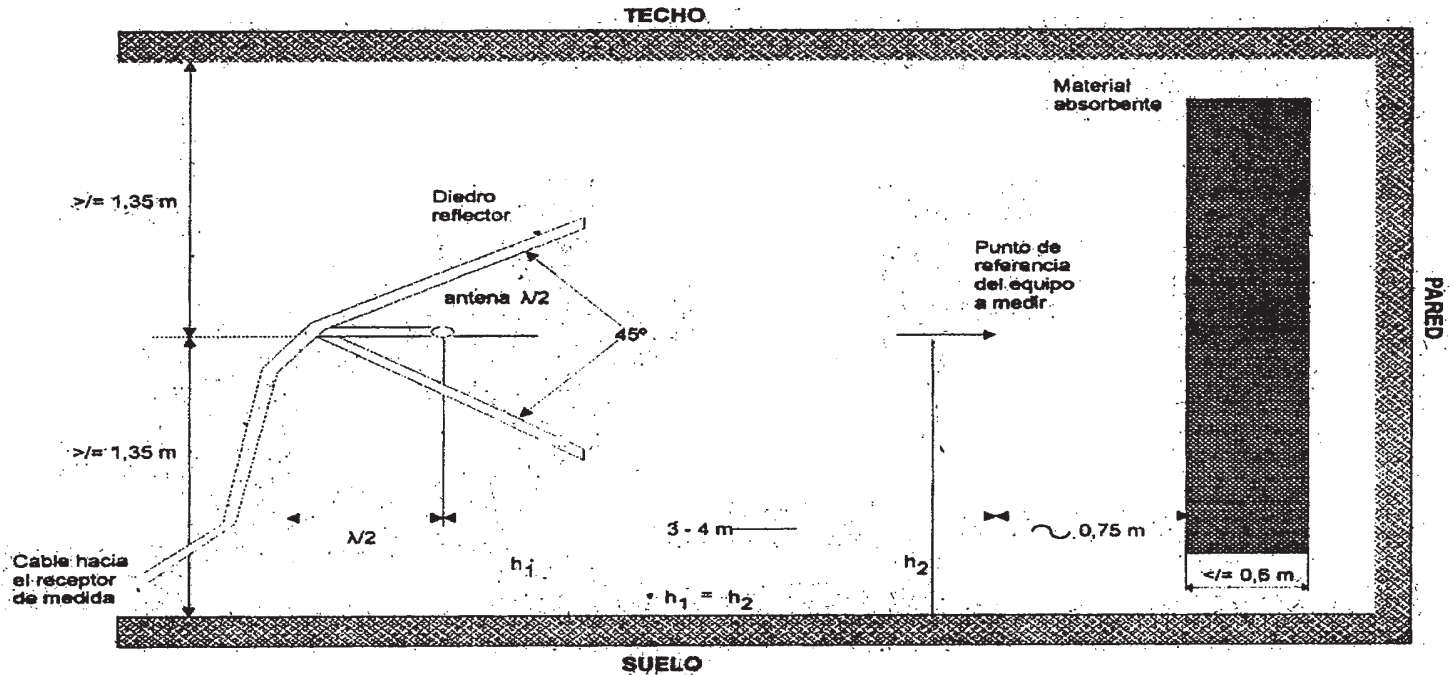
Figura 1: Disposición del recinto interior (caso de polarización horizontal)
