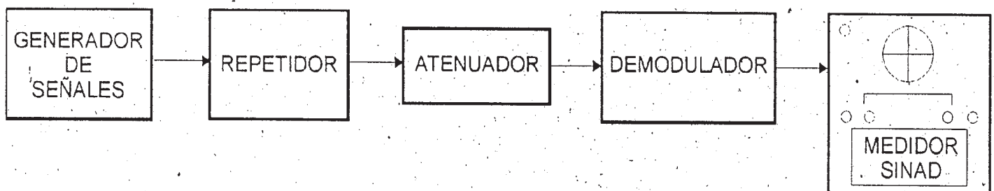
Figura 8: Montaje de medida de la distorsión de la banda de paso
