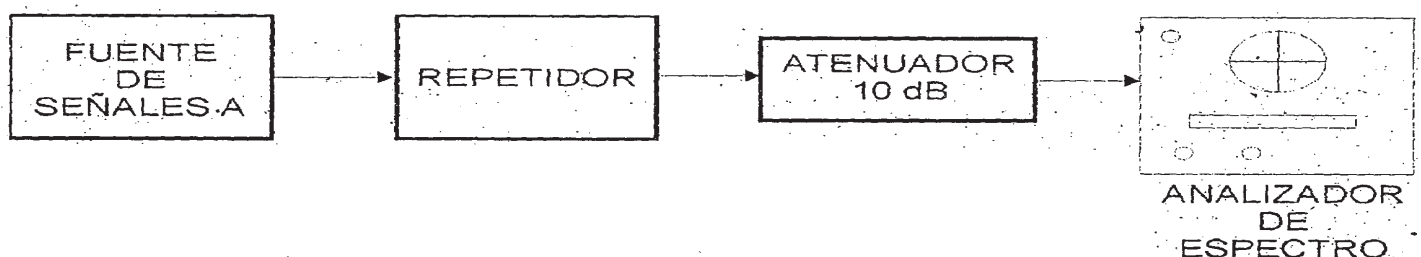
Figura 7: Montaje de medida de la potencia en el canal adyacente
