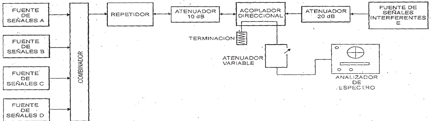
Figura 5: Montaje de medida para la atenuación de intermodulación (señal interferente en la salida)
