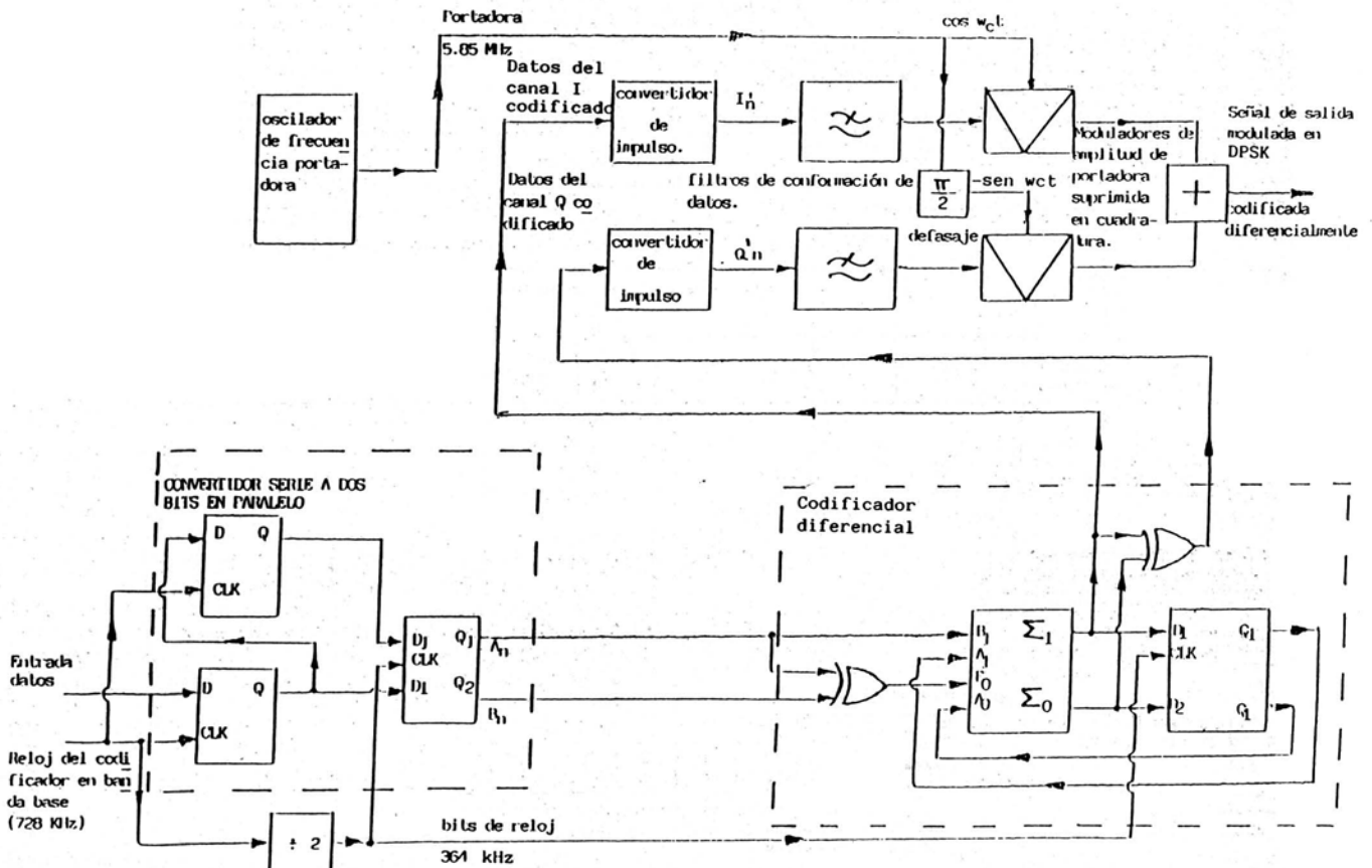
Fig. 5. Diagrama de bloques mostrando los procesos de codificación diferencial, conformación del espectro de señal-datos y modulación en el transmisor.
