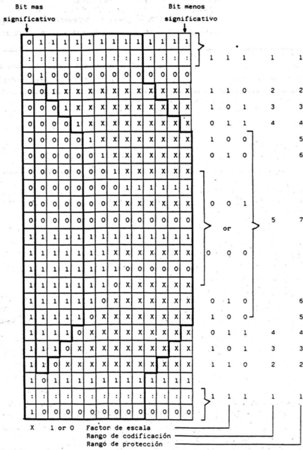
Fig. 2. Codificación de compresión-expansión de señales de sonido
