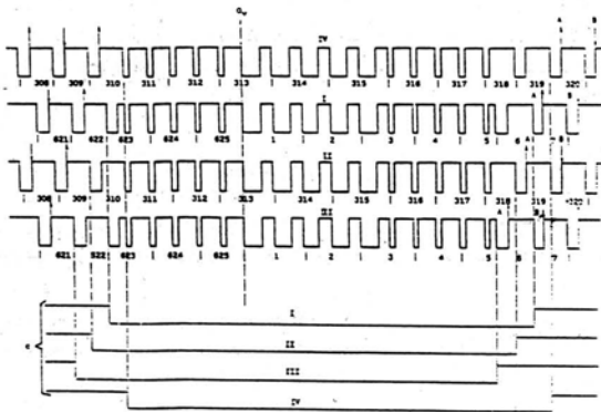
FIGURA 5 - Secuencia de supresión de la ráfaga
