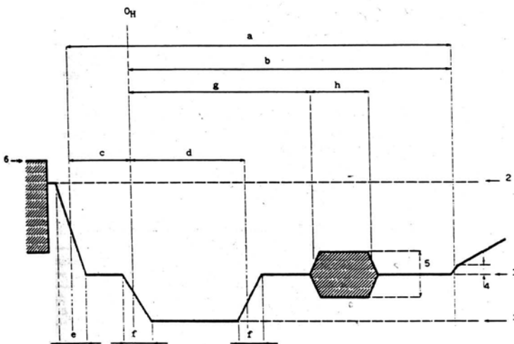
FIGURA 1 - Niveles de la señal compuesta y detalles de las señales de sincronismo de línea
