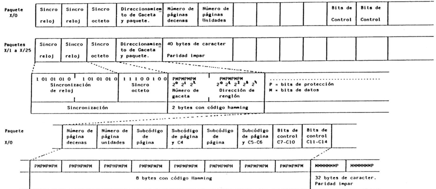
Formato de los paquetes X/0 a X/25
