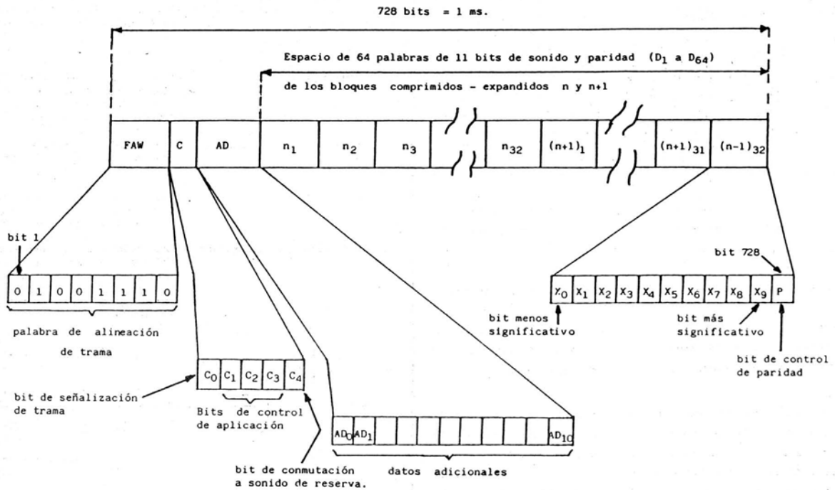
Fig. 1 (b) Estructura de la trama de 728 bits conteniendo una señal de sonido mono (antes de la transposición).
