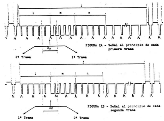
FIGURA 2 - Detalle de las señales de sincronismo de trama
