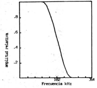
Fig. 4 (b) Respuesta de amplitud de los filtros de conformación de pulsos del conjunto transmisor y receptor ideal.
